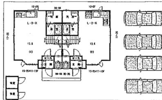
町道 1F平面図 ・ 配置図
