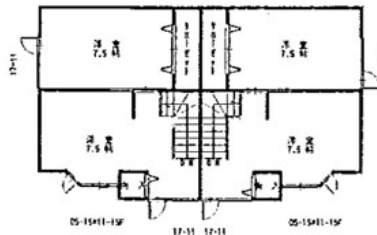
2F平面図
